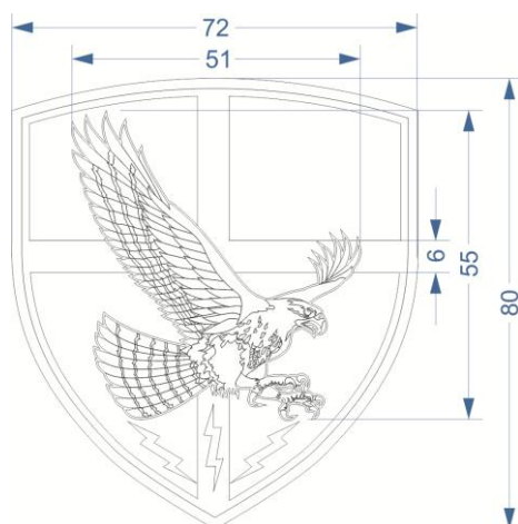
Слика 72. Димензије амблема батаљона за противтерористичка дејства Специјалне бригаде
